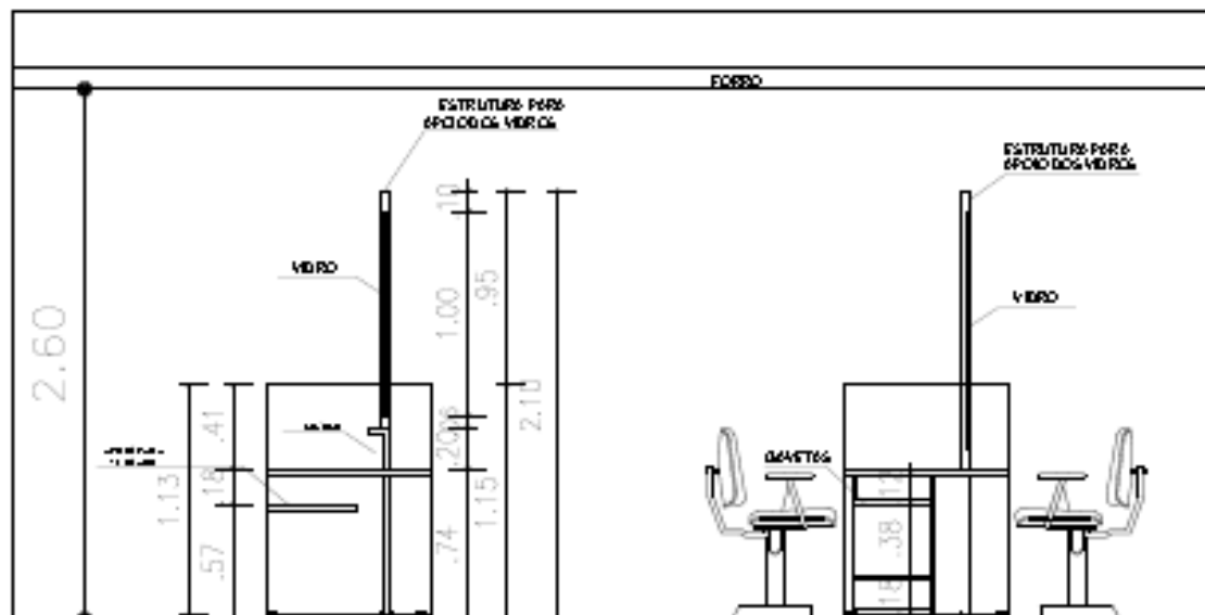
VISTA LATERAL
