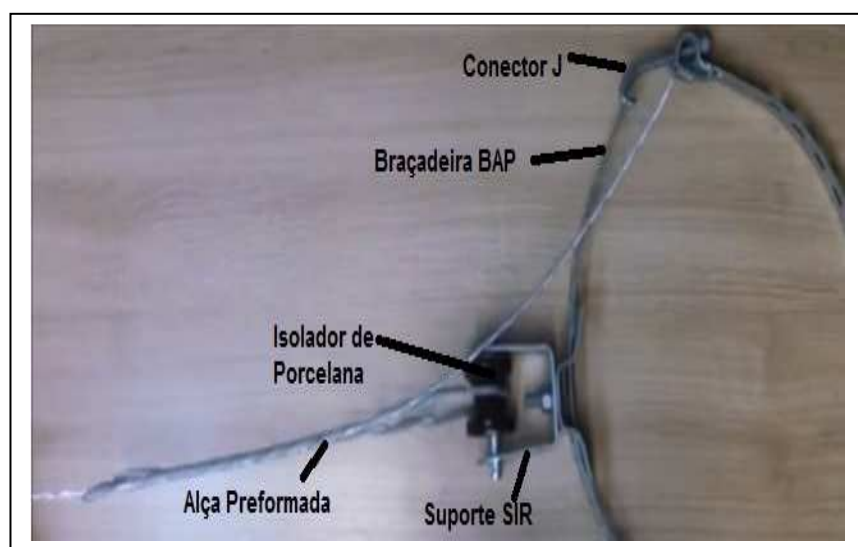
Figura XII – Conjunto de Ancoragem 02
