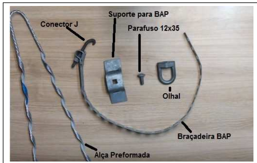
Figura XI – Conjunto de Ancoragem 01
