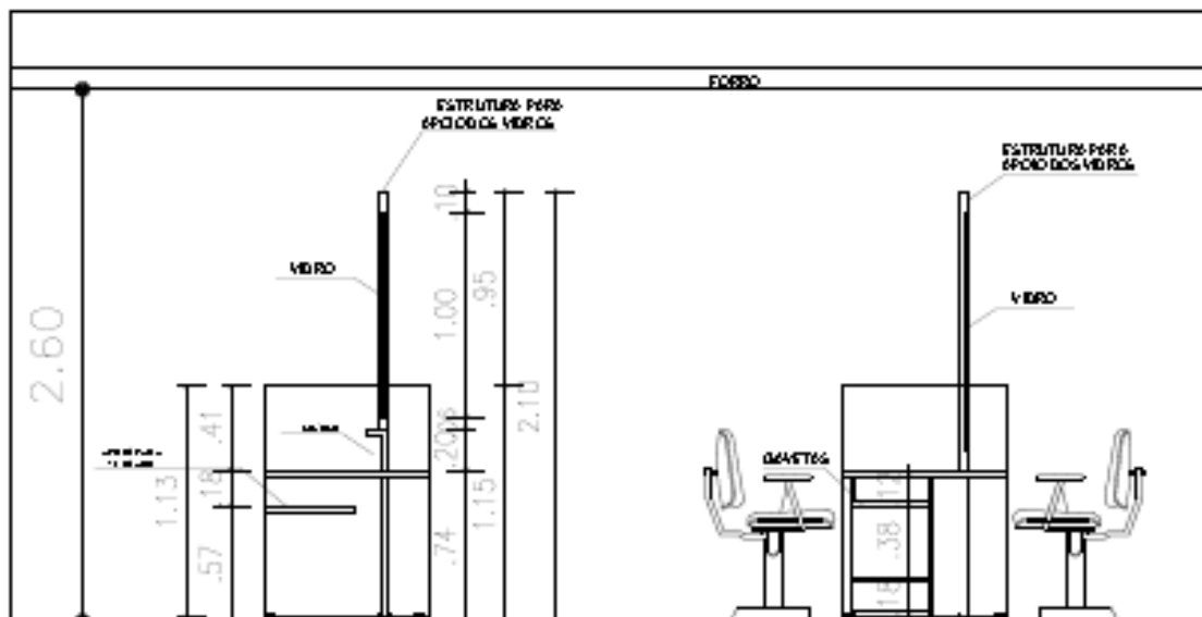
VISTA LATERAL
