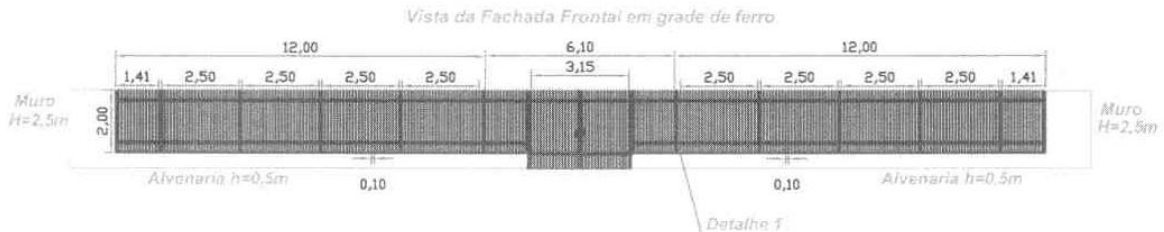
DESENHO 2: grades da sala de custódia
